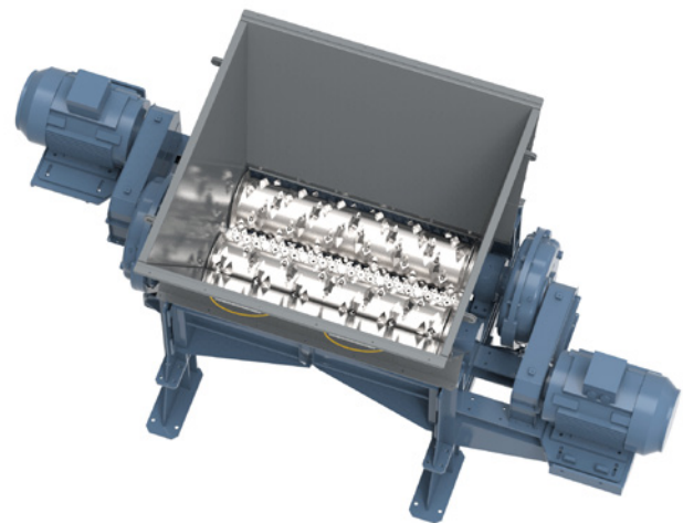
Abb.2: Draufsicht, mit Rotoren
