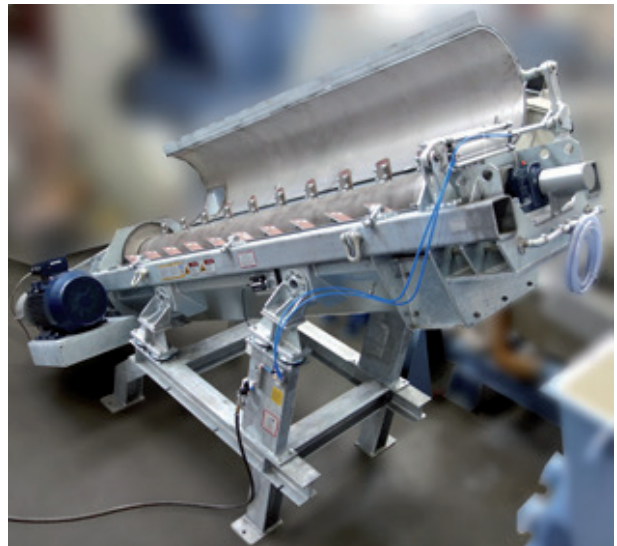
Abb. 9: Pneumatische Öffnung für Wartungszugang, Reduzierung von Stillstandszeiten
