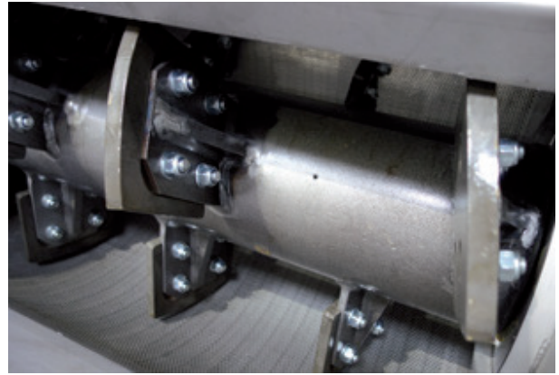
Abb. 8: Austauschbare Verschleißpaddel
